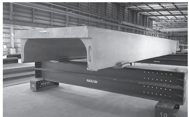
写真 - 9 脱型後の製品状況
