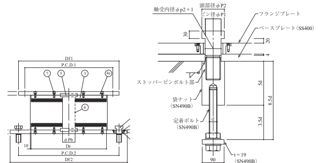
図 - 9 浮上り機構を有する免震装置詳細
