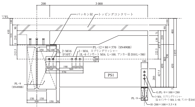
図 - 16 モックアップ組立図
