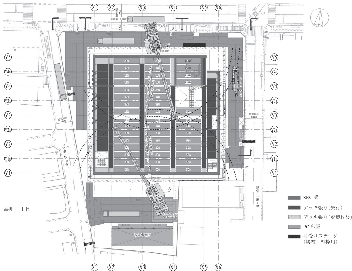
図-17 総合仮設計画図
