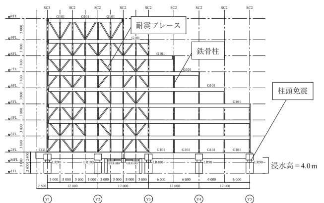
図 - 8 東面軸組図とブレース配置
