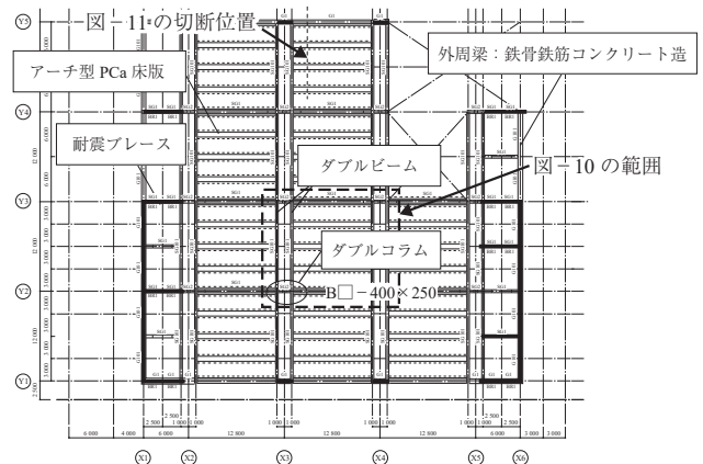
図 - 7 構造計画概要
