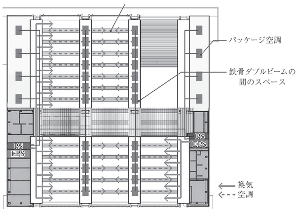
図-4 オフィスの空調計画
