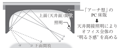
図-6 アーチ型PC床版の照明装置としての利用
