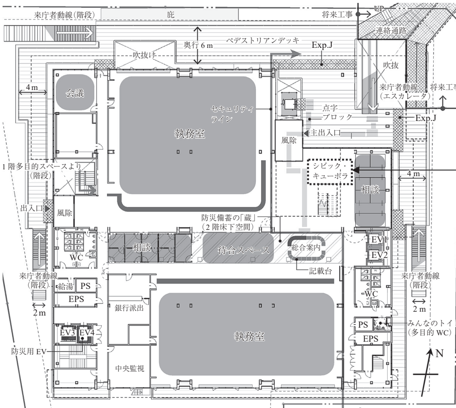
図-3 2階平面図
