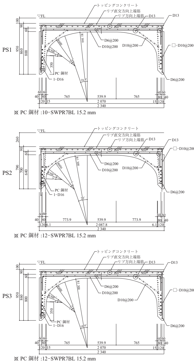
図 - 13 PC 床版断面形状
