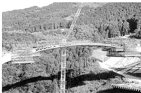
写真-7 コンクリート巻立て施工状況
