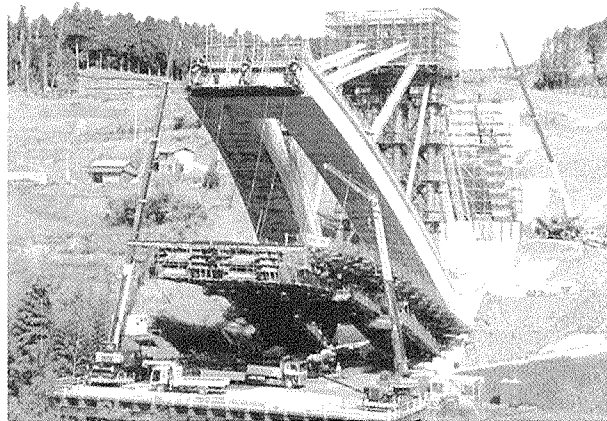
写真 - 5 吊り支保工解体状況
