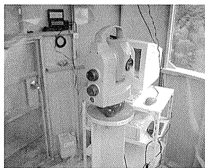
写真-3 自動視準トータルステーション
