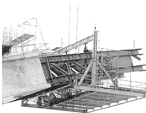
写真 - 6 メラン架設用作業足場
