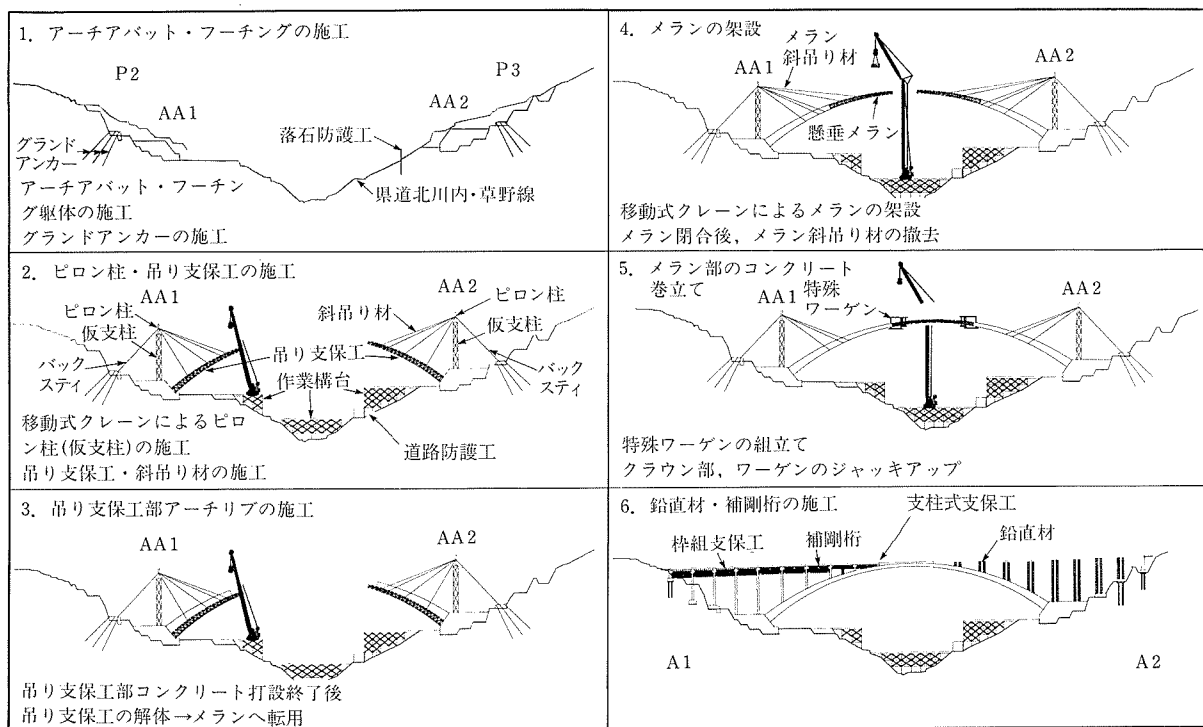
図 - 2 施工手順
