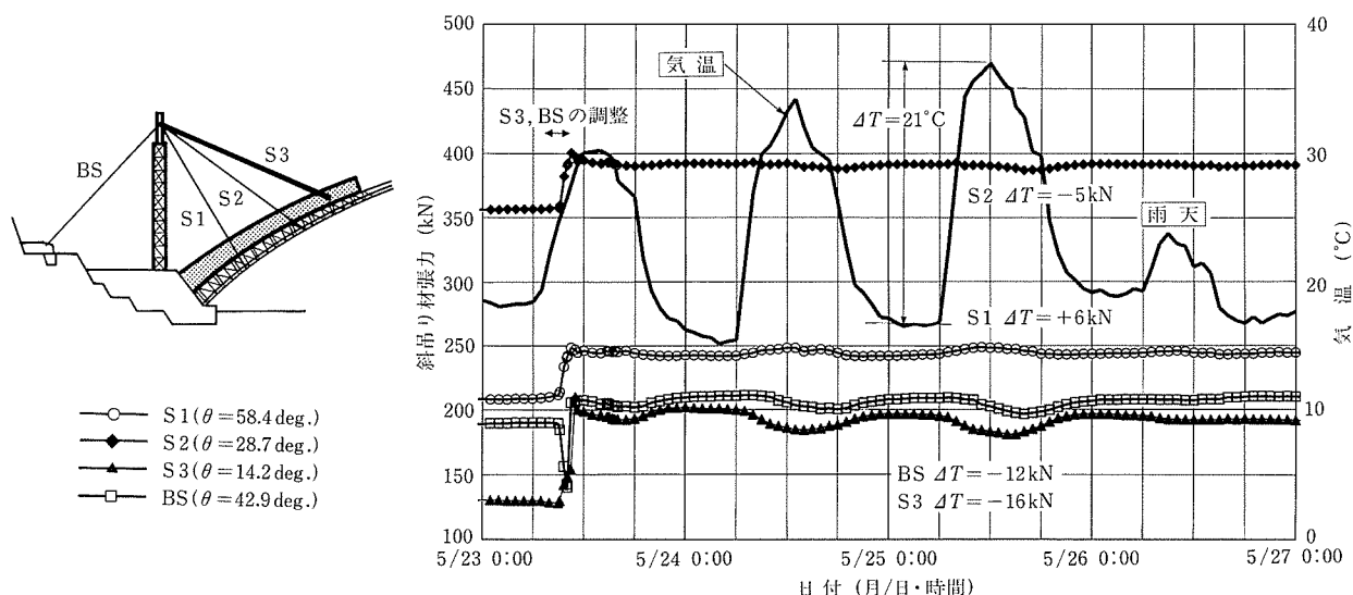
図-8 吊り支保工施工時における斜吊り材張力変
