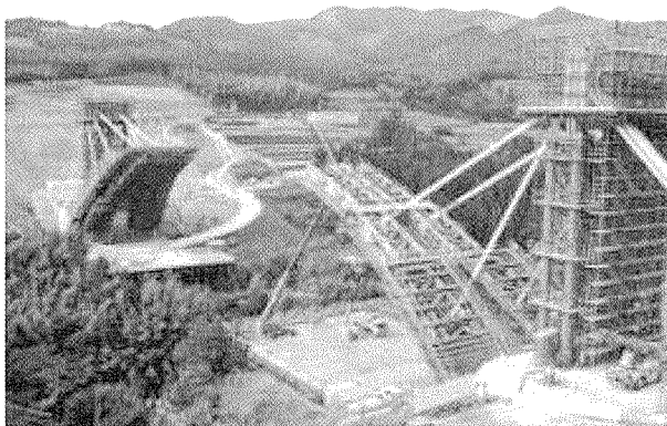
写真 - 4 吊り支保工
